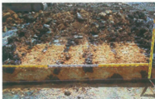
写真-5 反転後の状況 (1段耕ブラウ)
