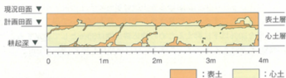
図-1 レーザーブラウ性能試験における反転状況
